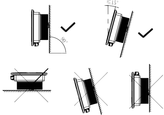
Abb. 5.1 Installationsschema
