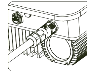
Abb 6.4 AC-Schnellanschluss-Schema
