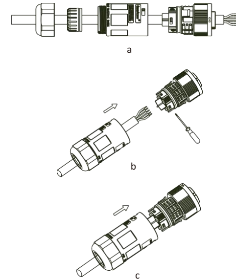
Abb 6.2 AC Ausgangsschalterschema
