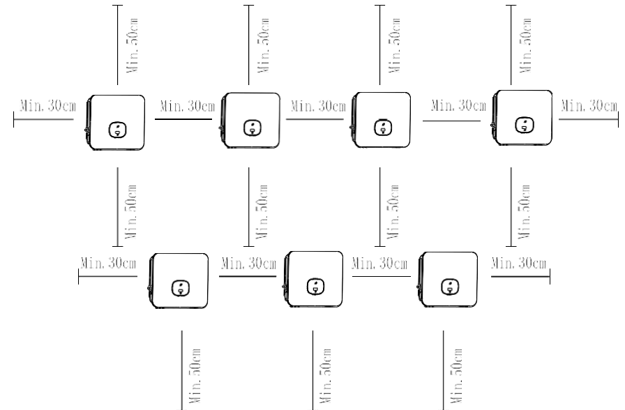
Abb. 5.3 Installationsdimensionen mehrerer Wechselrichter
