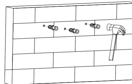
Abb 5.8 Schematische Darstellung der Wandmontage
