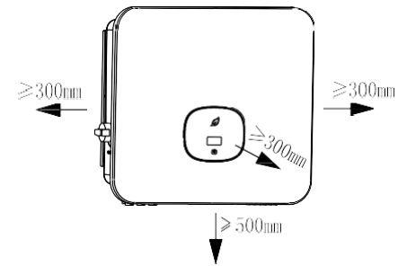
Abb. 5.2 Installationsdimensionen des Wechselrichters
