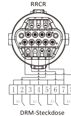
Abb 6.18 Wechselrichter – RRCR-Verbindung
