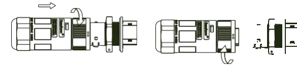
Abb 6.3 Anschlussschema der AC-Klemme
